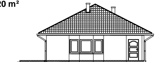
ELEWACJA POŁUDNIOWA
